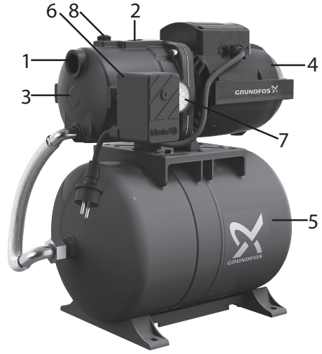
Рис. 2 Внешний вид установки JPA PT
